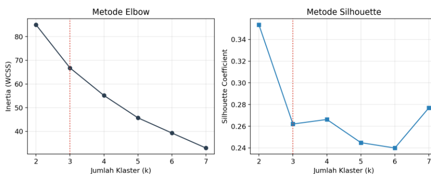
Gambar 1. Grafik Metode Elbow (kiri) dan Grafik Metode Silhouette (kanan)
